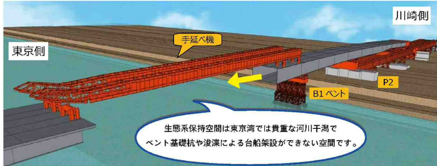
送出し架設イメージ図
